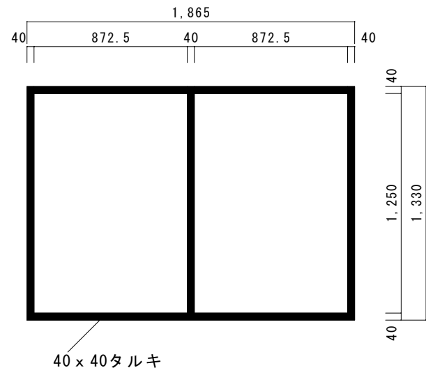
タルキ伏図〔上部〕 1/30
