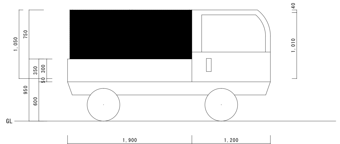
側面 1/30
