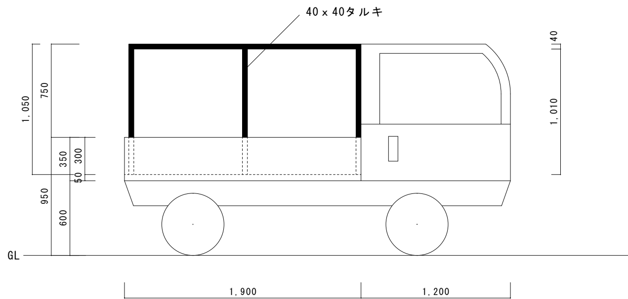
タルキ伏図〔側面〕 1/30
